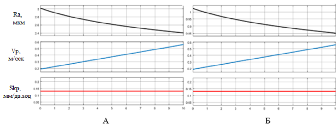
Рис. 2. График зависимости шероховатости поверхности от скорости резания при постоянной круговой подаче
