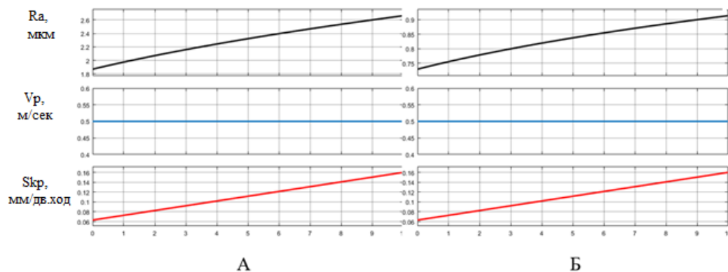
Рис. 1. График зависимости шероховатости поверхности от круговой подачи при постоянной скорости резания
